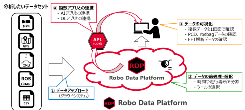
RoboDataPlatform データ分析フローイメージ
