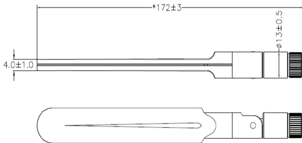
図2.5-5 LTE Antenna
