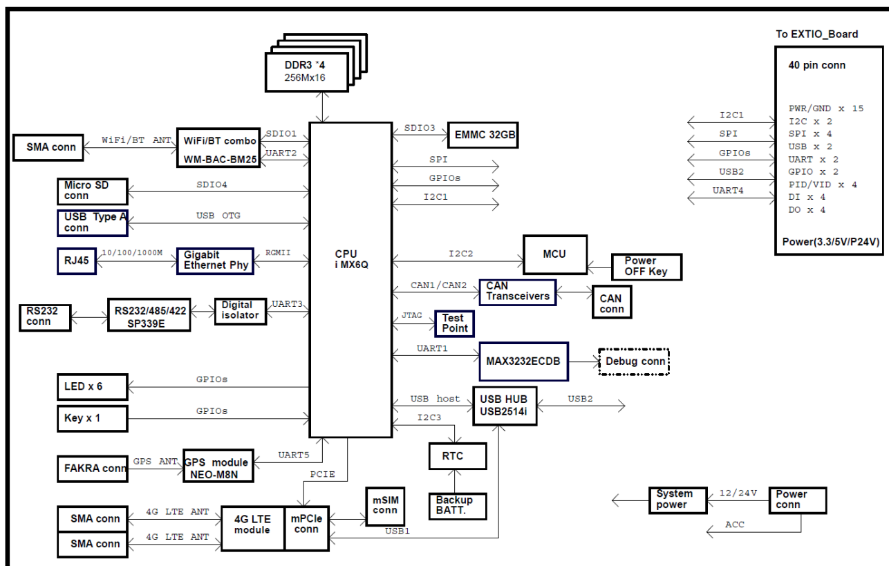
図2.3-1 ブロック図
