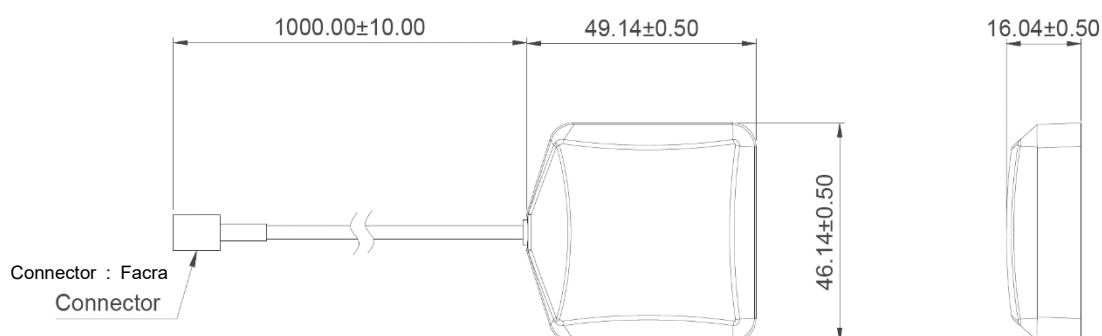
図2.5-7 GNSS Antenna
