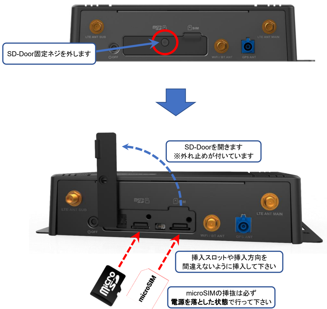
図3.1-1 microSIM および microSDの挿入
