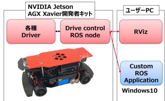
RoboCar 1/10X システム構成
